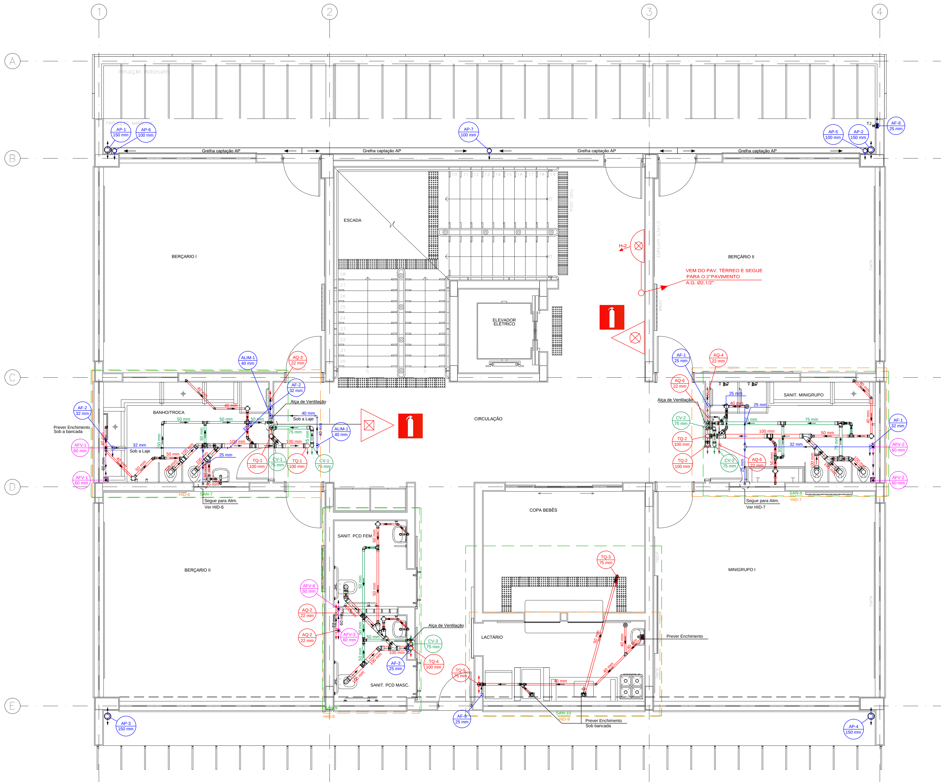
PLANTA BAIXA - PRIMEIRO PAVIMENTO Escala 1:50
